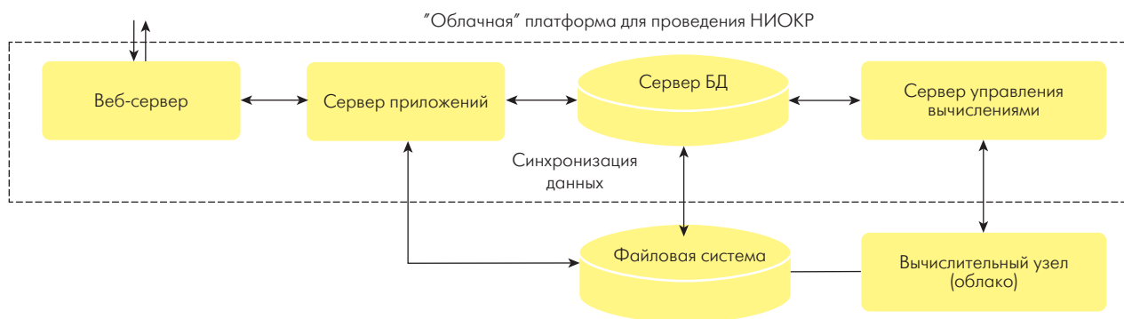
Рис.2. Архитектура верхнего уровня R&D Paas
